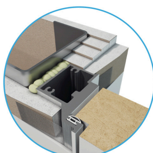
MARCO DE PUERTA DE ALUMINIO / INTERNO - LADRILLO / TABIQUE CARTÓN YESO
